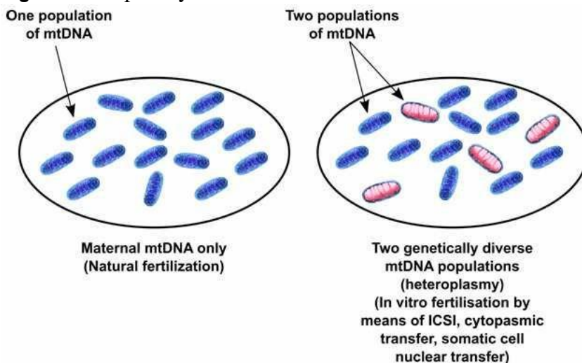
Fig. 9. Heteroplasmy
